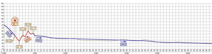
ESQUEMA HIDRÁULICO - SOLUÇÃO A Escala: H=1:20 000; V=1:1000
